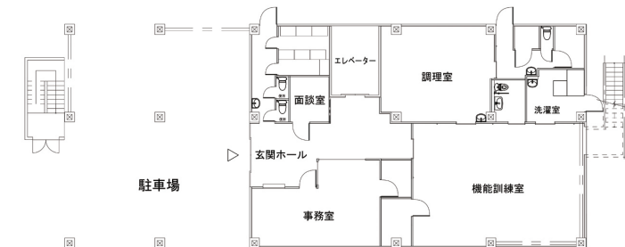
1階平面図
